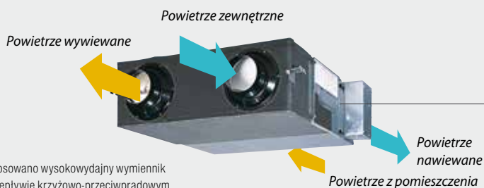
Wymiennik innego producenta (wymiennik krzyżowy)
